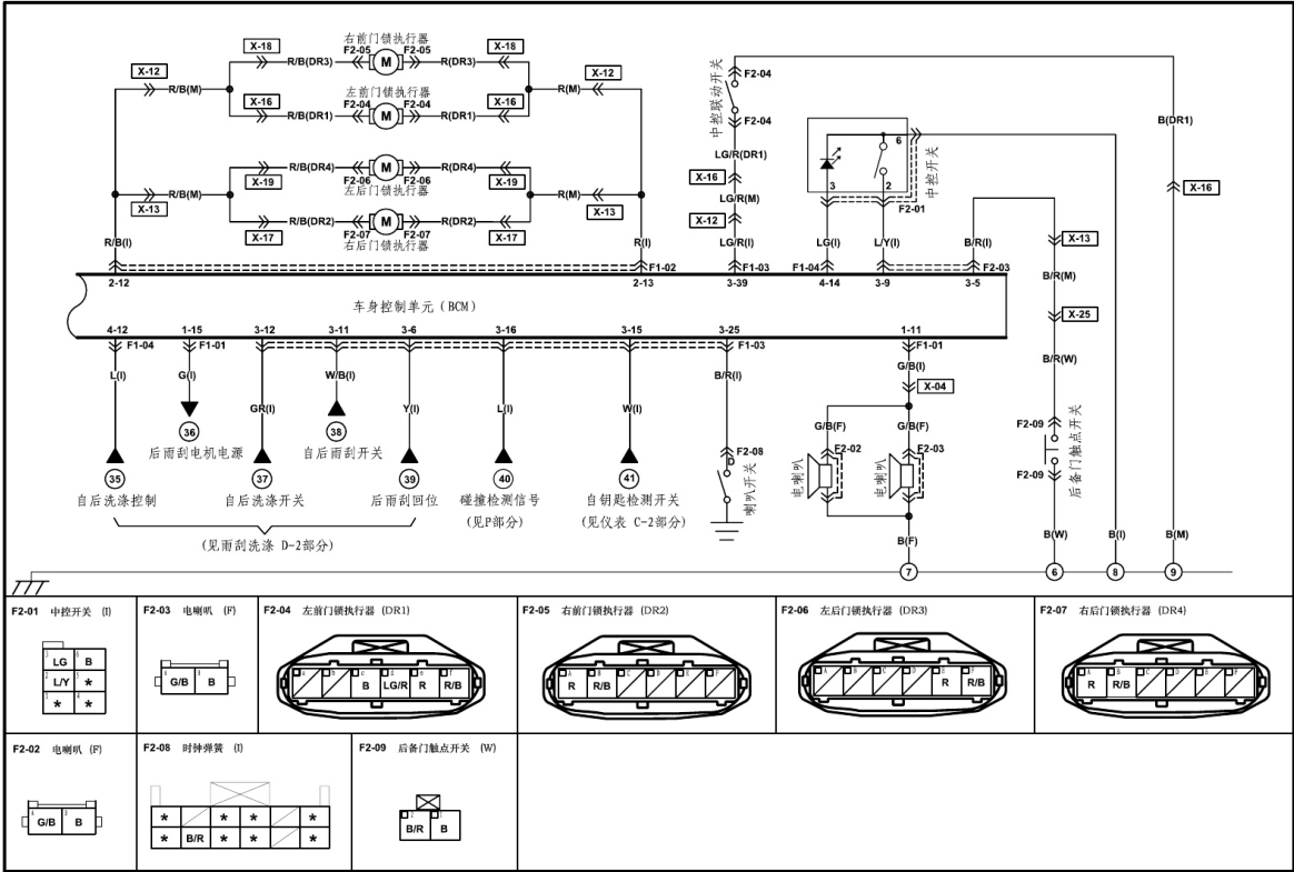
BCM控制单元（后雨刮洗涤/喇叭/门锁电机）
