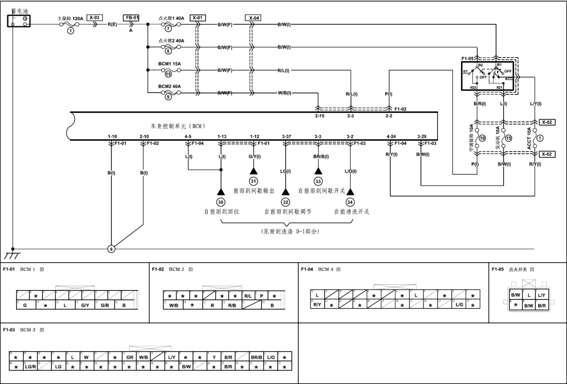
BCM控制单元 (电源/前雨刮洗涤)
